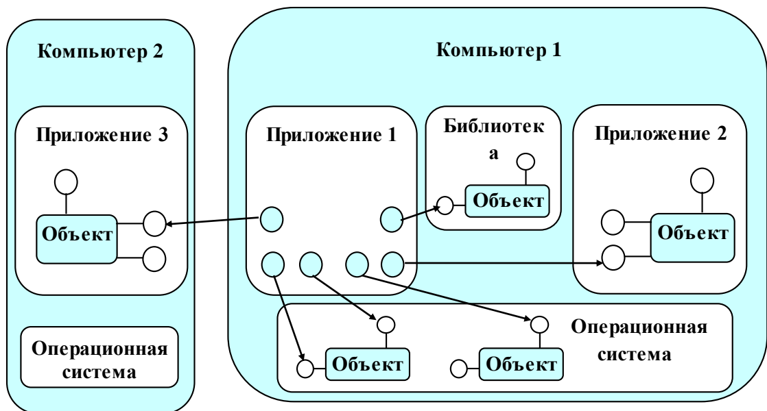
Рисунок А.4 – Компонентный подход. Технология COM
