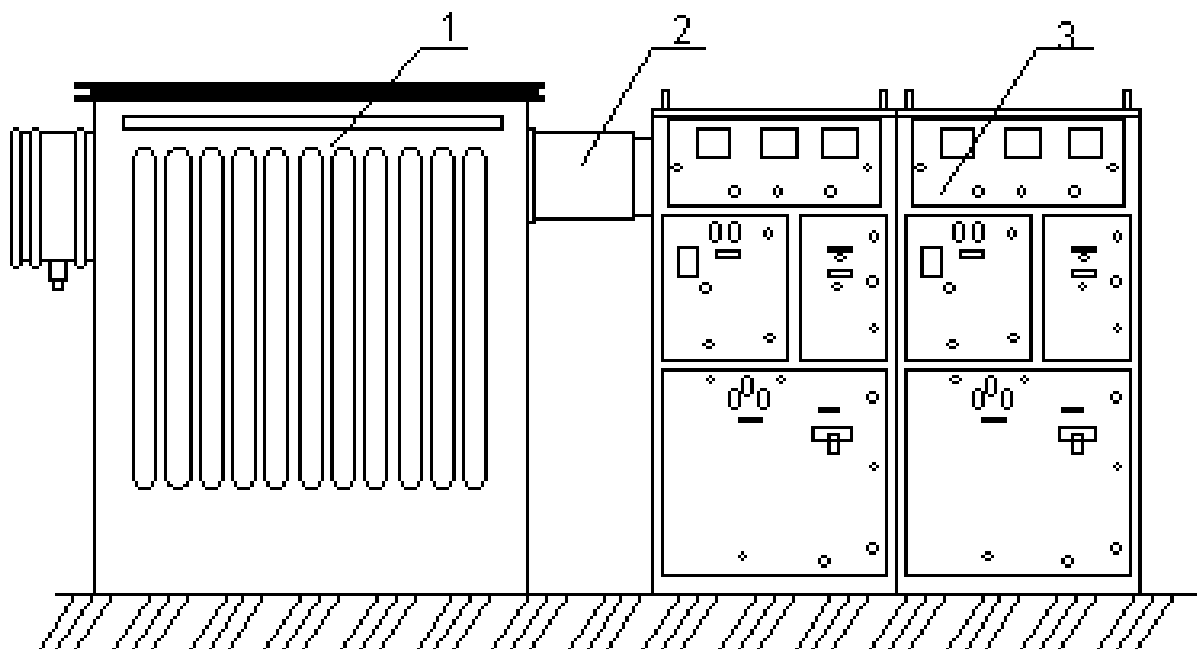
8.1 сурет – Ішке орнатылатын КТҚС
