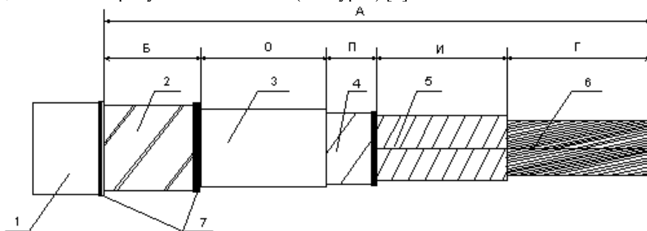
1 – сыртқы қабат; 2 – сауыт; 3 – қабықша; 4 – белдеулік оқшаулама; 5 – тарамның оқшауламасы; 6 – кабель тарамы; 7 – белтартпа; А, Б, И, О, П, Г – тарқатудың өлшемдері.
