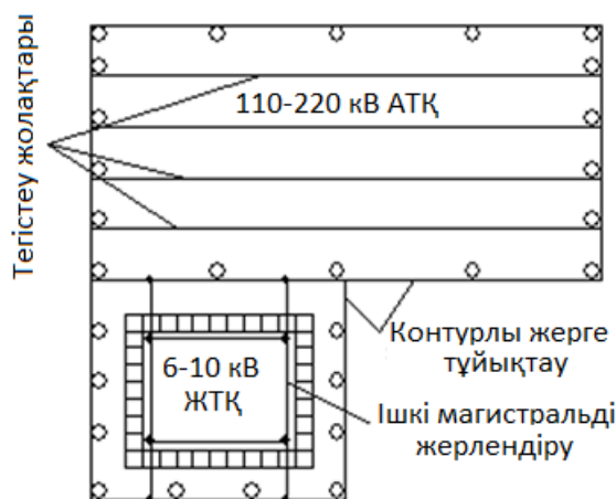
7.1 сурет – Қосалқы стансаның жерлендіру контуры
