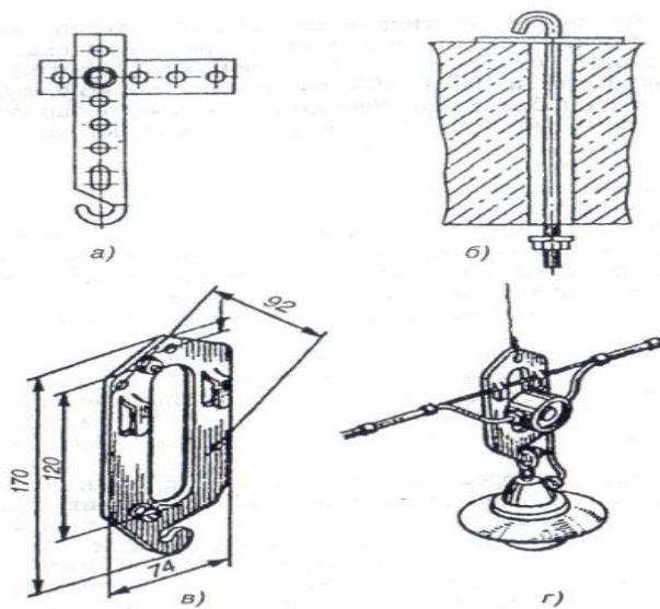
11.1 сурет – Шамдарды орналастыру үшін конструктивті элементтер
