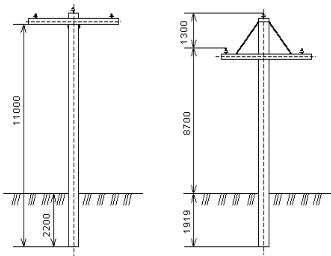
10.2 сурет- ВЛ-10 кВ аралық бағаналары.
