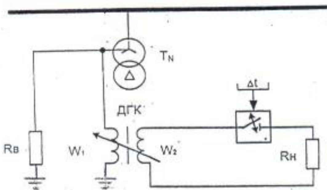
14.1 сурет – 6 – 35 кВ электр тораптарының бейтарап режимдері
