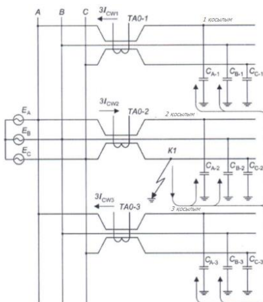
14.3 сурет - Бір фазалы жерге тұйықталу кезіндегі токтың бағыты мен желісінің сұлбасы
