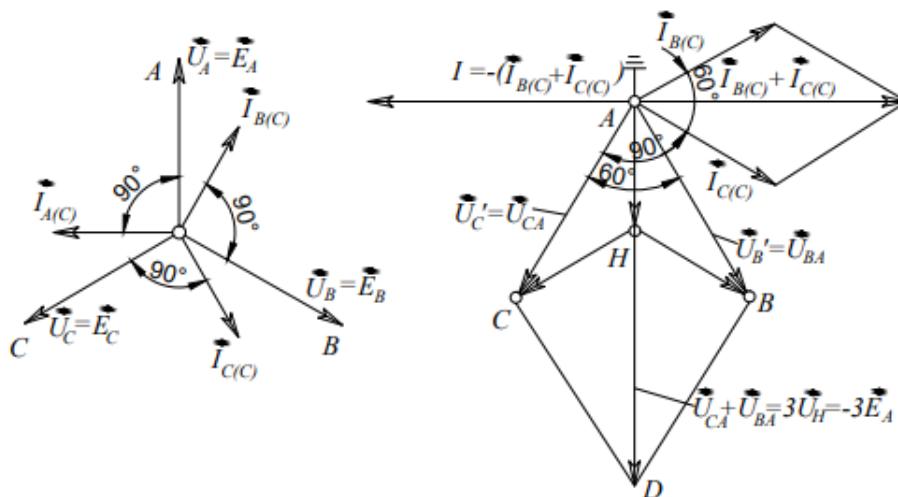
14.4 сурет- Векторлық диаграммалар қалыпты режимде және бір фазалы жерге тұйықталған кезде
