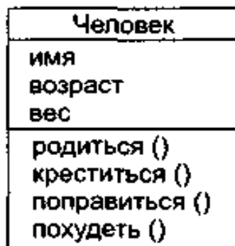
Рисунок 3.1 - Отображение класса
