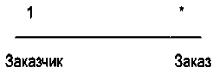
Рисунок 3.2 - Ассоциация
