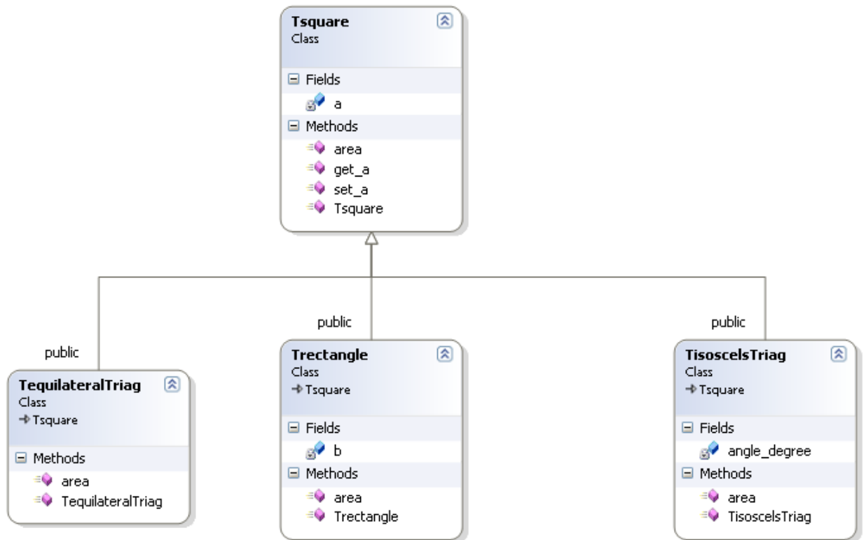
Рисунок 3.4 – Диаграмма классов
